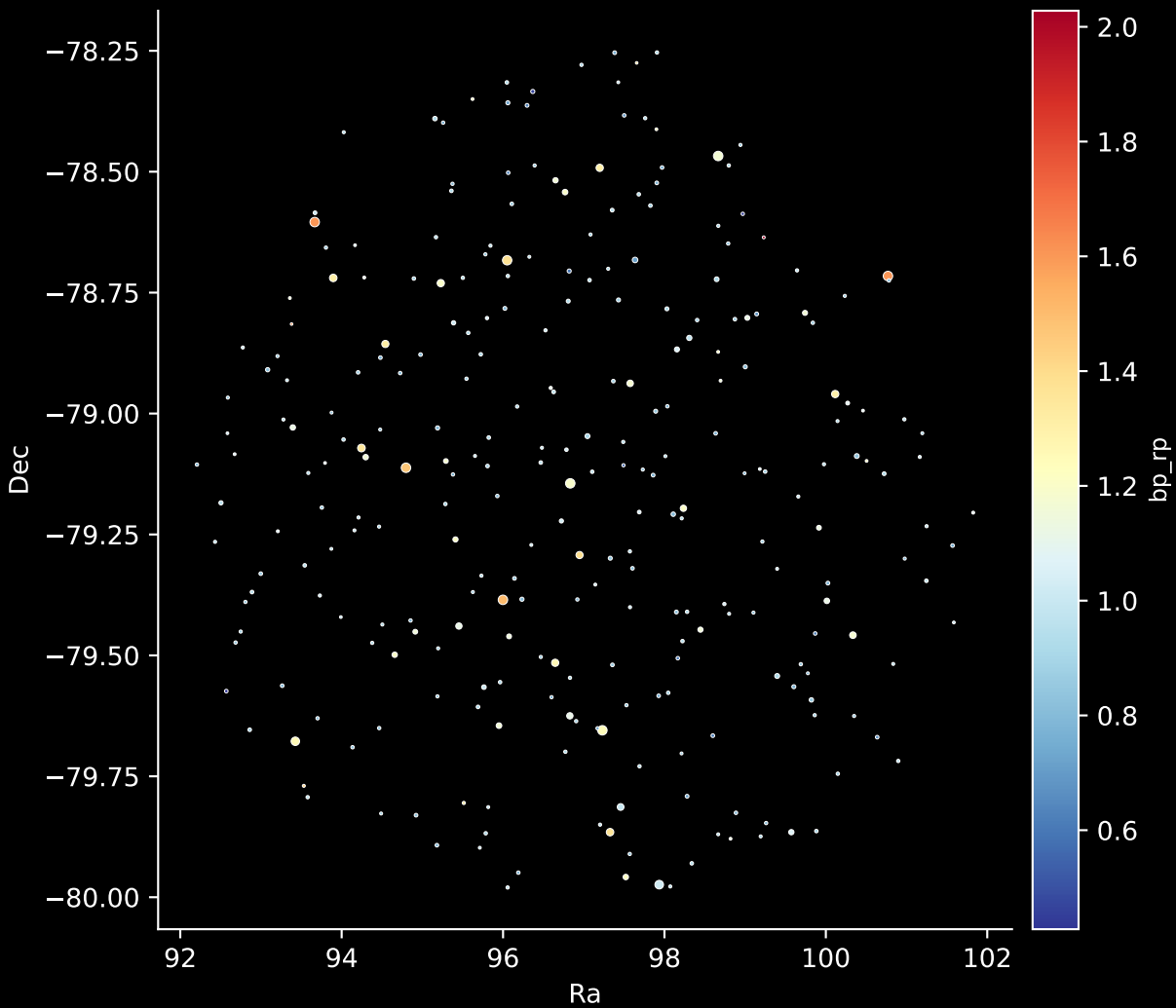
GALAH DR4 Field: [321] Stars: 279
