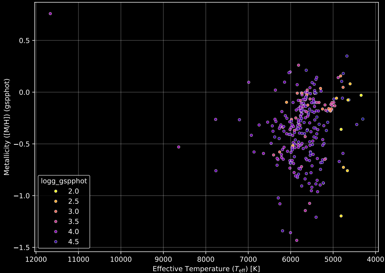
GALAH DR4 Field: [321] Stellar Population Parameters (n= 279)
